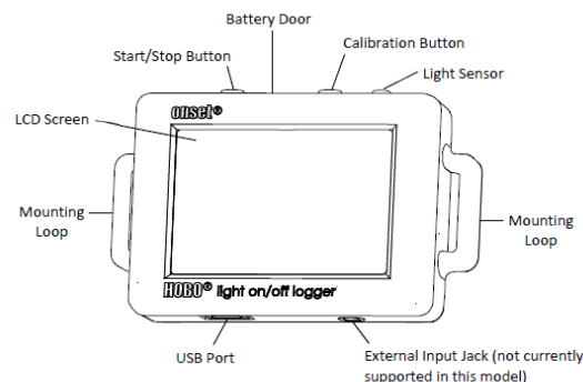
ロガー各部名称
