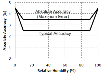
グラフ B: 湿度精度
