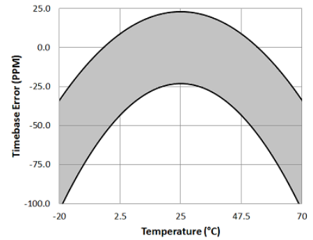
グラフ C: 時間精度
