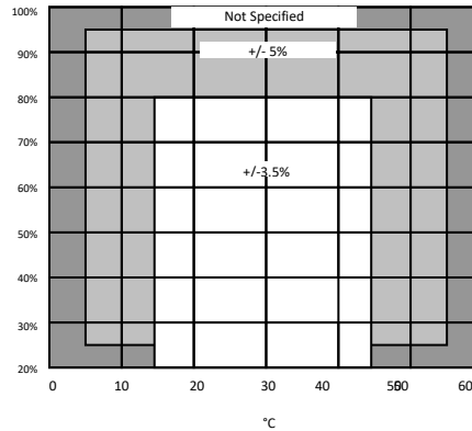
グラフ B: 温度精度
