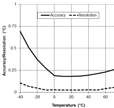
グラフ A: 温度精度と分解能
