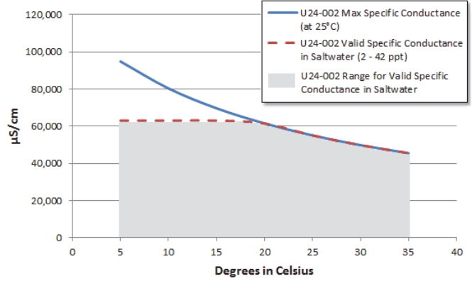
Plot B 電気伝導率範囲 (温度補償後)
