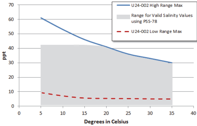
Plot A 塩分範囲
